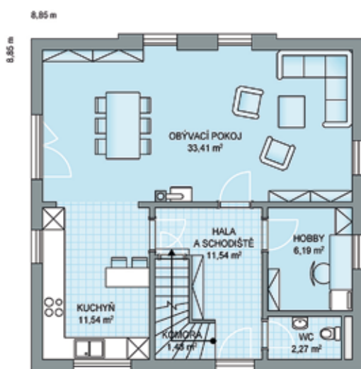
Přízemí
