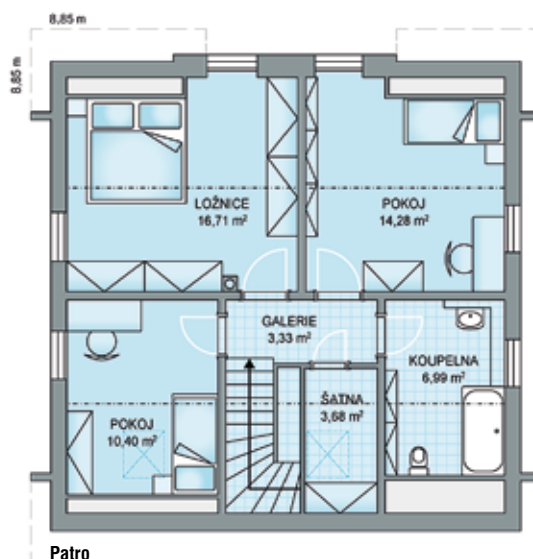
Patro
